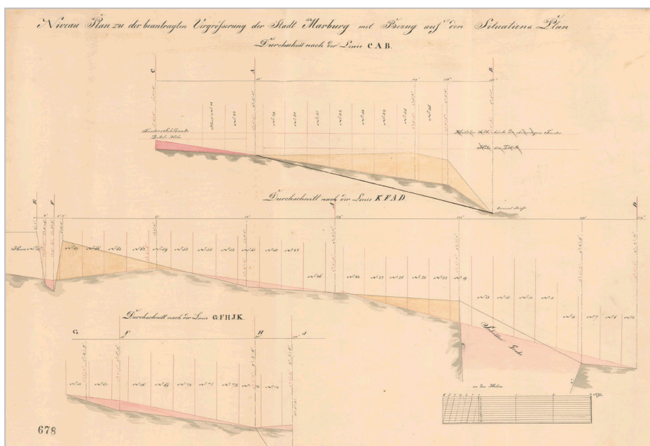
Nivojski načrt za povečanje mesta Maribor, 1846 (StLA, KA Marburg, Fasz. 11/2, K. 29, 1836–1848, gradbeni spis 2538/1847, fol. 678r)
