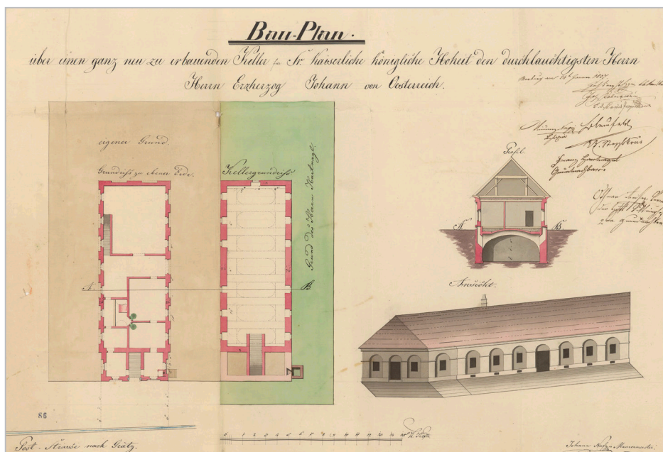
Johann Georg Nafz, Načrt za klet nadvojvode Janeza na Partizanski cesti 15/Cankarjevi ulici 1, 1836 (StLA, StLA, KA Marburg, Fasz. 11/2, K. 29, 1836–1848, gradbeni spis 2538/1847, fol. 86r)
