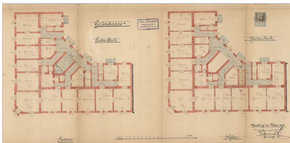
Franz Derwuschek, Načrt za gradnjo večstanovanjske najemniške hiše v lasti stotnika Josefa Matasića in soproge Juliane. Tlorisa prvega in drugega nadstropja, 1897 (PAM, fond Uprava za gradnje in regulacijo Maribora 1840–1963, Maistrova ulica 17, gradbeni spisi in gradbena dokumentacija, str. 1a)
