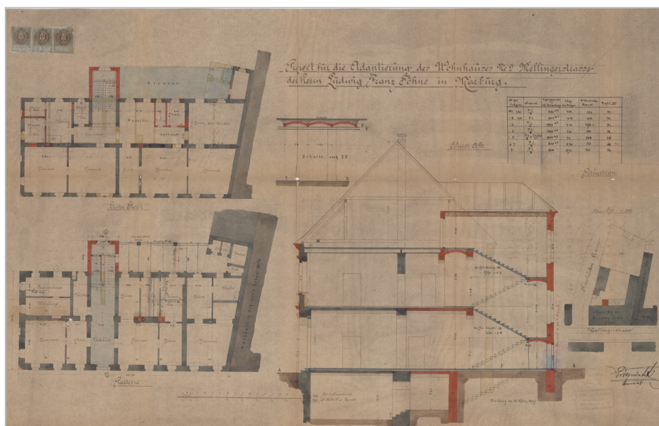
Franz Derwuschek, Načrt za prezidavo stanovanjske hiše v lasti Ludwiga Franza in sinov, 1897 (PAM, fond Uprava za gradnje in regulacijo Maribora 1840–1963, Meljska cesta 11, gradbeni spisi in gradbena dokumentacija, str. 2a)
