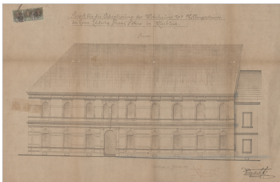
Franz Derwuschek, Načrt za ureditev južnega pročelja stanovanjske hiše v lasti Ludwiga Franza in sinov, 1897 (PAM, fond Uprava za gradnje in regulacijo Maribora 1840–1963, Meljska cesta 11, gradbeni spisi in gradbena dokumentacija, str. 3a)
