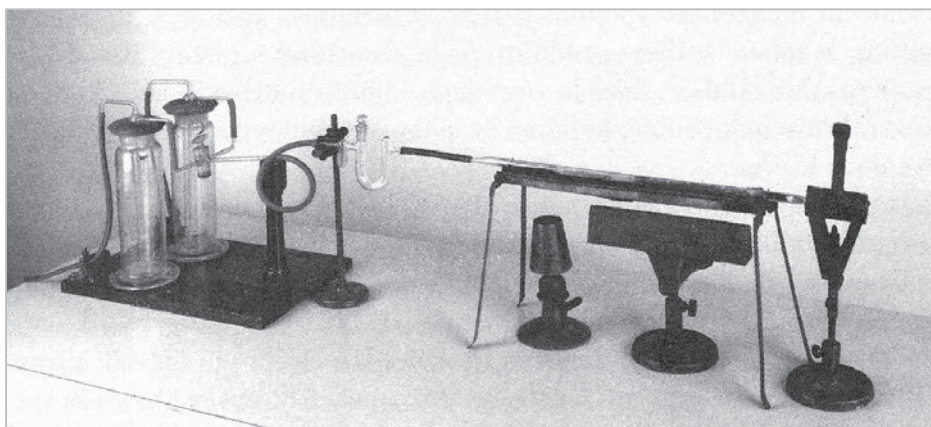
Del originalne Preglove aparature za mikroanalizo ogljika in vodika v organskih spojinah, ki jo je avtor podaril Univerzi v Ljubljani (vir: Modrijan založba, d. o. o., foto: Tomaž Lunder)
