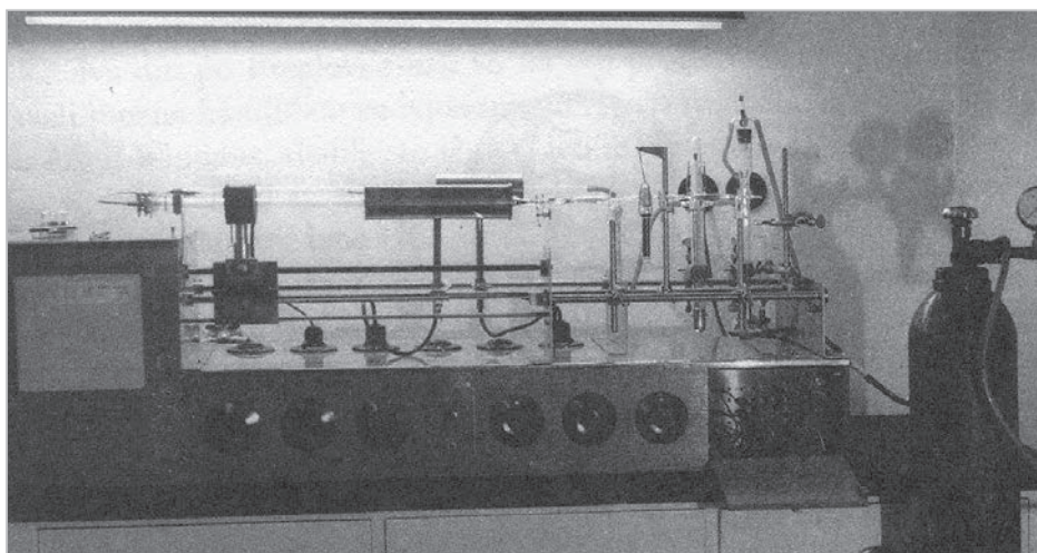
Preglova aparatura za mikroanalizo ogljika in vodika v organskih spojinah v Preglovem laboratoriju Univerze v Grazu. Aparatura je posodobljena in ima ohranjene vse bistvene sestavne dele prvotne Preglove aparature (foto: akad. Miha Tišler)
